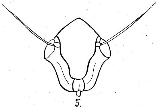
Sabimamorpha speciosissima n. sp.
