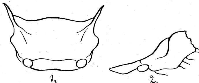
Ledra kosempoensis n. sp. Kopf u. Pronotum von vorn.
